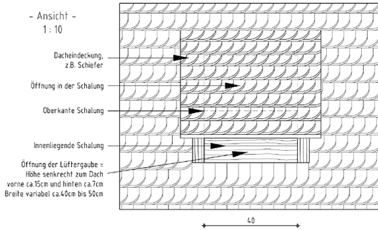
Schleppgaube Frontansicht
