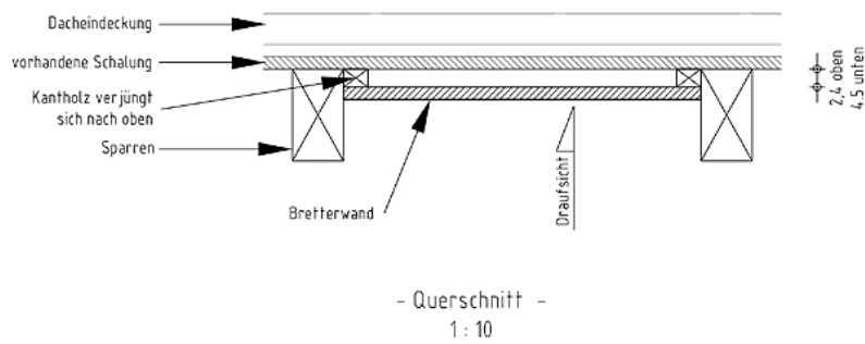
Spaltenquartier im Sparrenfeld Querschnitt
