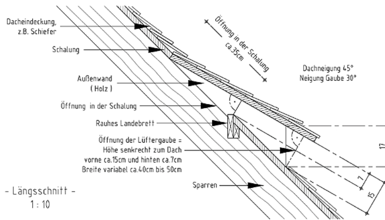
Schleppgaube Längsschnitt
